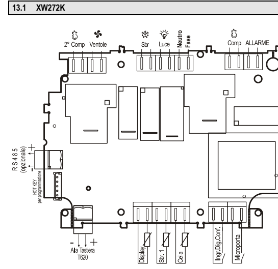
Tastiera T620
